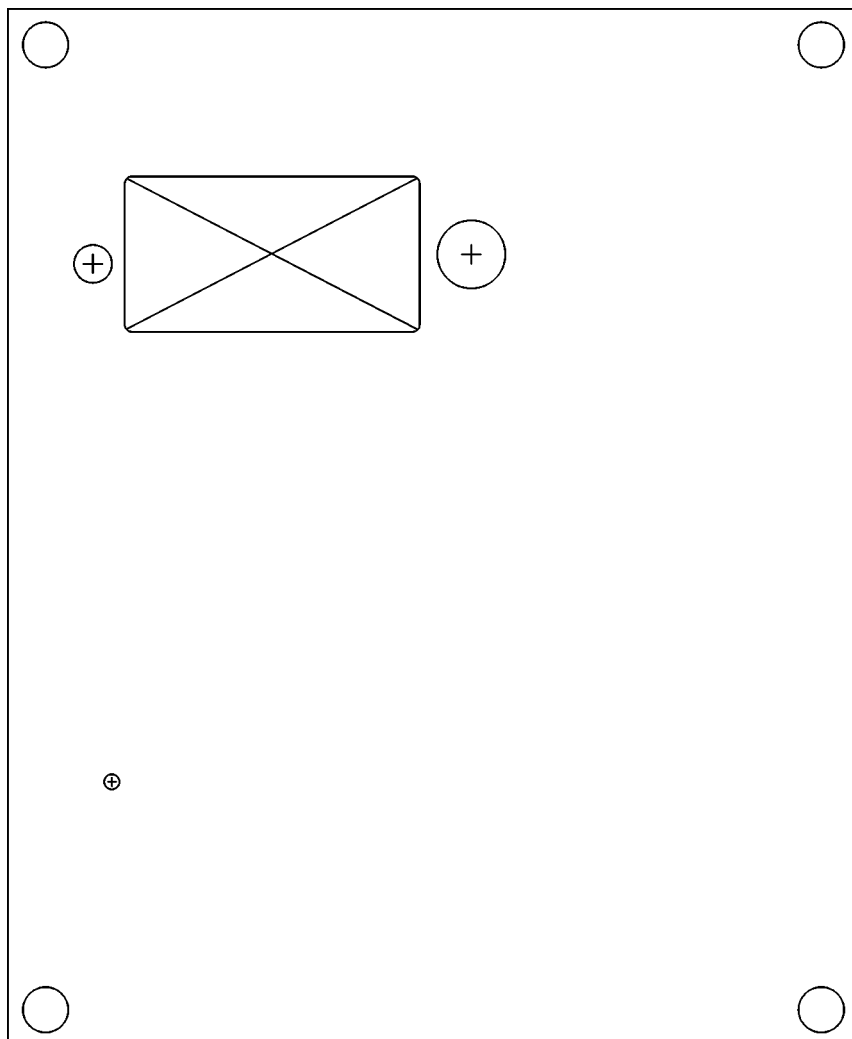
Vrtací šablona krabičky Vrtací šablona.tif
